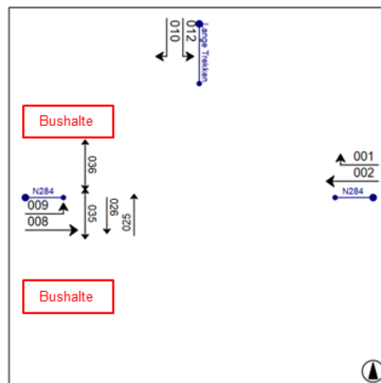
Figuur 17 Kruispuntvormgeving (schematisch)
