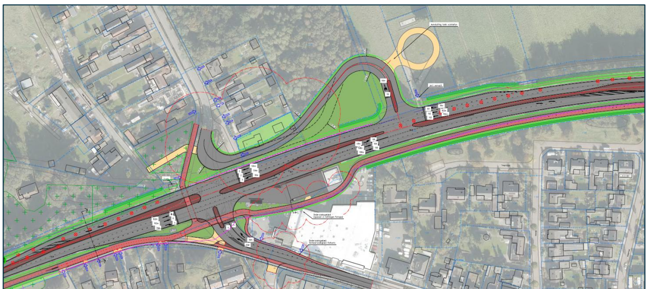
Figuur 20 Conceptschets kruispunt N284 – Castersedijk
