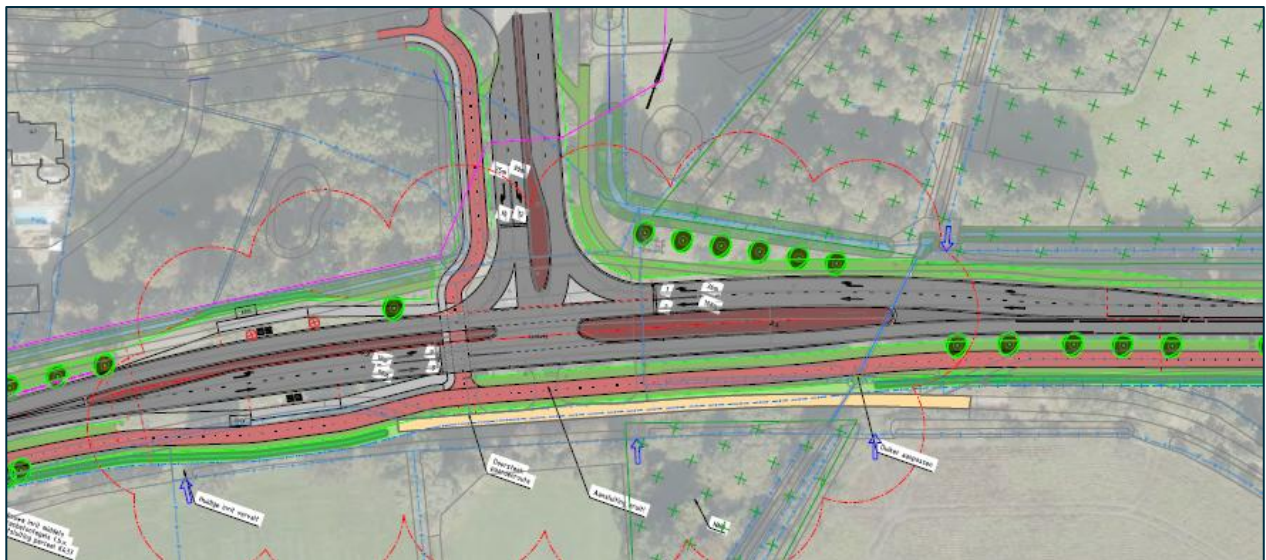
Figuur 18 Conceptschets kruispunt N284 – Lange Trekken
