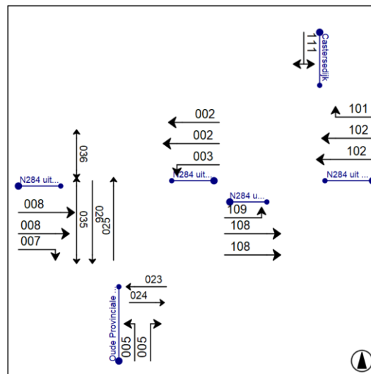
Figuur 19 Kruispuntvormgeving (schematisch)
