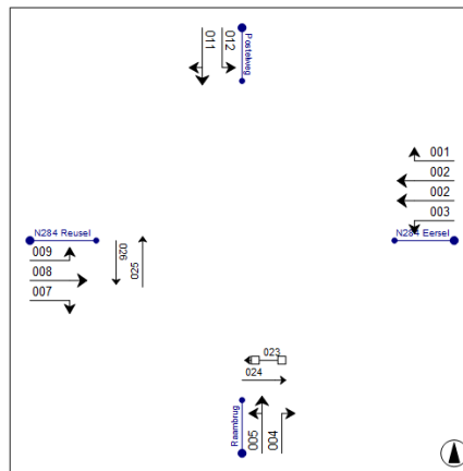
Figuur 13 Kruispuntvormgeving (schematisch)
