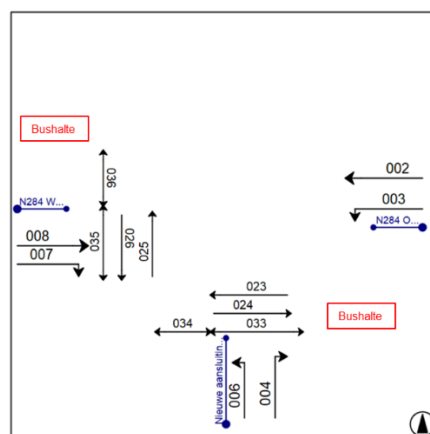
Figuur 11 Kruispuntvormgeving (schematisch)
