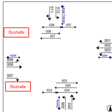
Figuur 15 Kruispuntvormgeving (schematisch)
