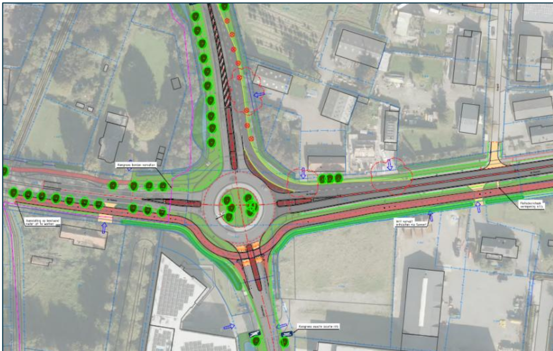
Figuur 10 Conceptschets kruispunt De Hoeven - N284
