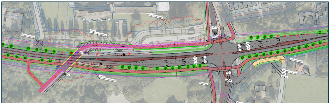
Figuur 16 Conceptschets kruispunt N284 – Europalaan
