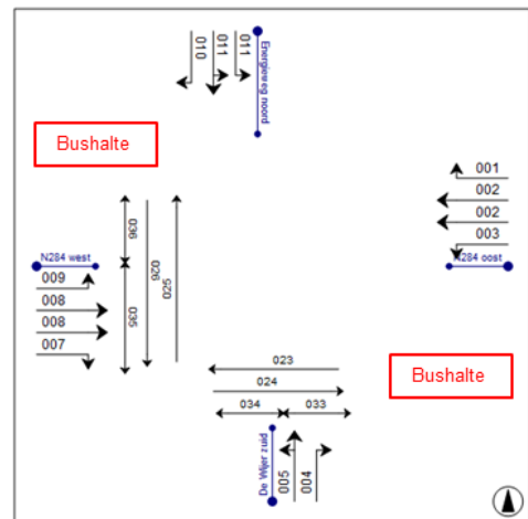
Figuur 21 Kruispuntvormgeving (schematisch)
