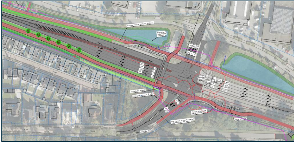
Figuur 22 Conceptschets kruispunt N284 – De Wijer
