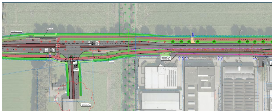
Figuur 12 Conceptschets kruispunt N284 – De Sleutel (nieuwe aansluiting)
