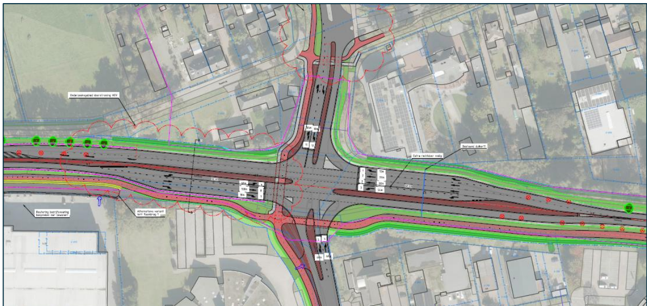
Figuur 14 Conceptschets kruispunt N284 – Raambrug
